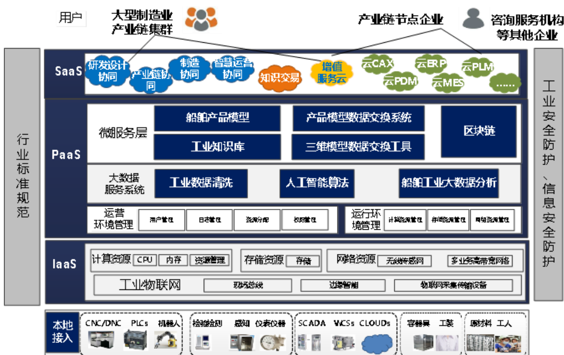
船舶工业智能运营平台架构图
